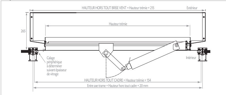
Coupe B-B
