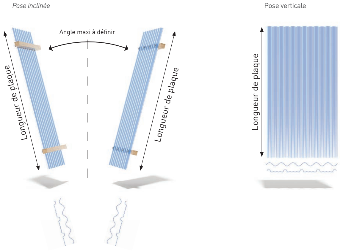
Ventilation: principe de pose protection d'isolant
