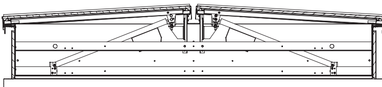
Tetracoif DoE en position d'attente
