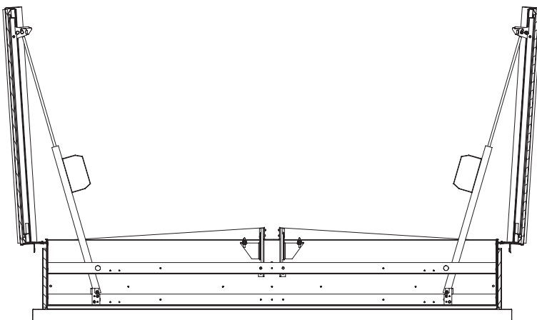
Tetracoif DoE en position de sécurité
