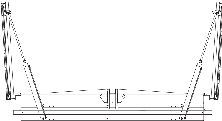
Tetracoif DoP Eco en position de sécurité - Ouverture 90°
