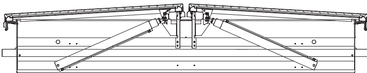
Tetracoif DoP Eco en position d'attente
