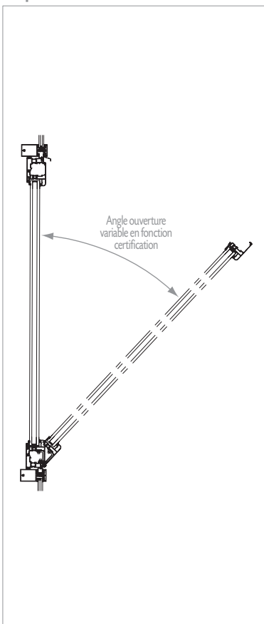
Coupes verticales
