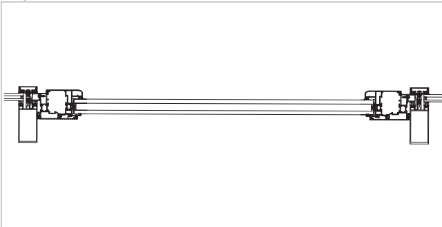
Coupes horizontales
